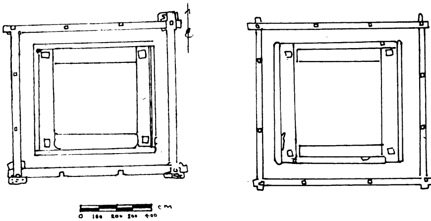
සැලසුම් 01-02- මාරස්සන අම්බලම හා කන්දෙවෙල පුරාණ අම්බලමේ බිම් සැලසුම් (මූලාශ්‍රය :- පානතේවාහැට ගවේෂණ වාර්තාව, 2009)
